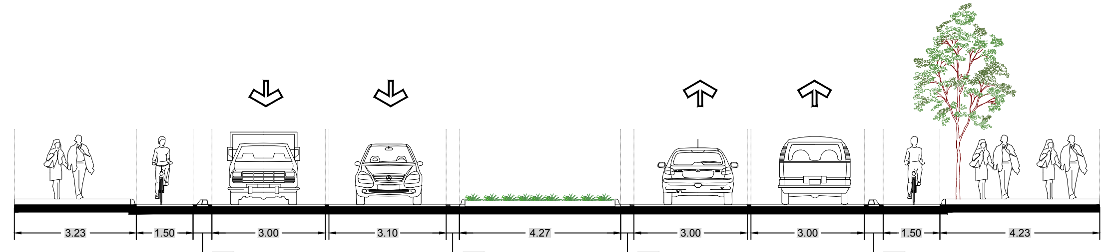
SECCIÓN DE CADENAMIENTO 1+340.00
