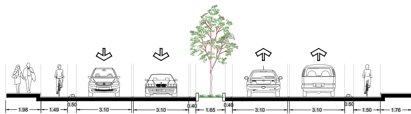
SECCIÓN DE CADENAMIENTO 2+220.00
