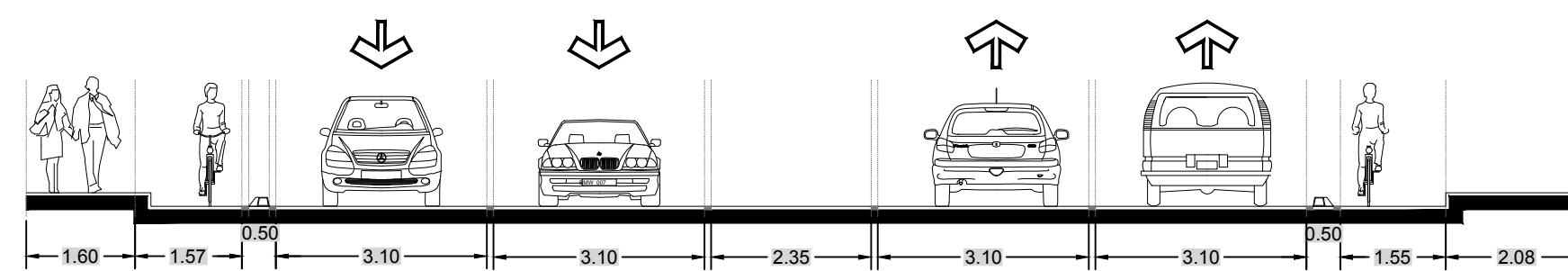
SECCIÓN DE CADENAMIENTO 2+320.00
