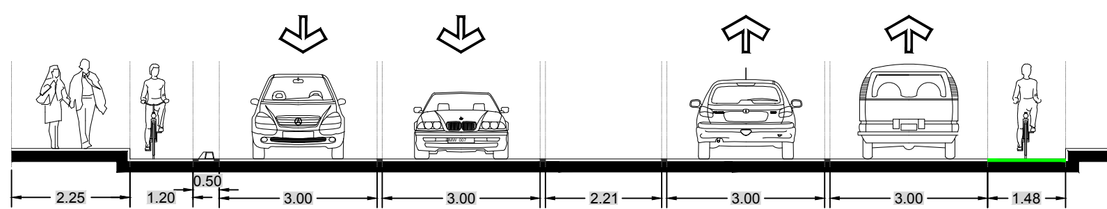
SECCIÓN DE CADENAMIENTO 2+900.00
