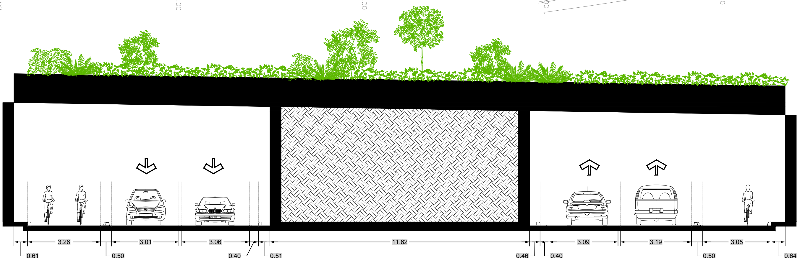
SECCIÓN DE CADENAMIENTO 1+100.00
