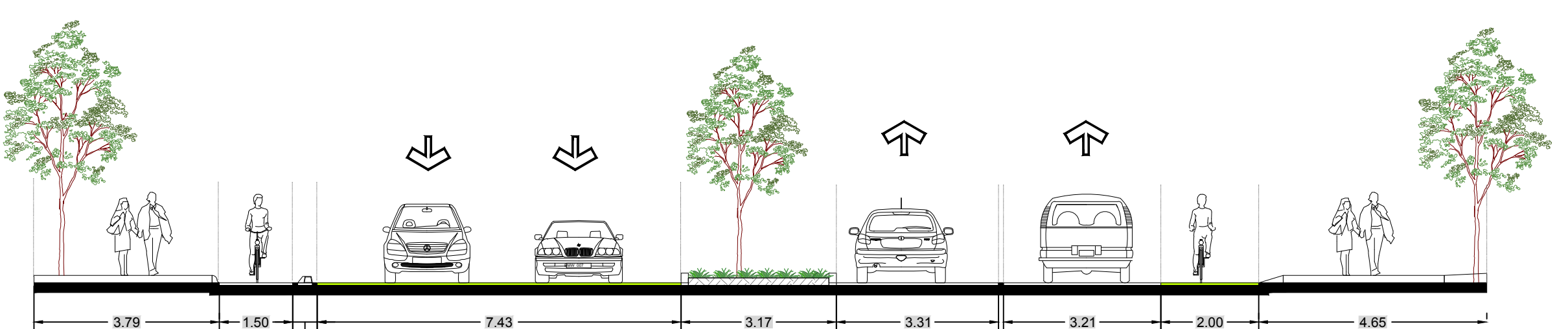
SECCIÓN DE CADENAMIENTO 1+900.00
