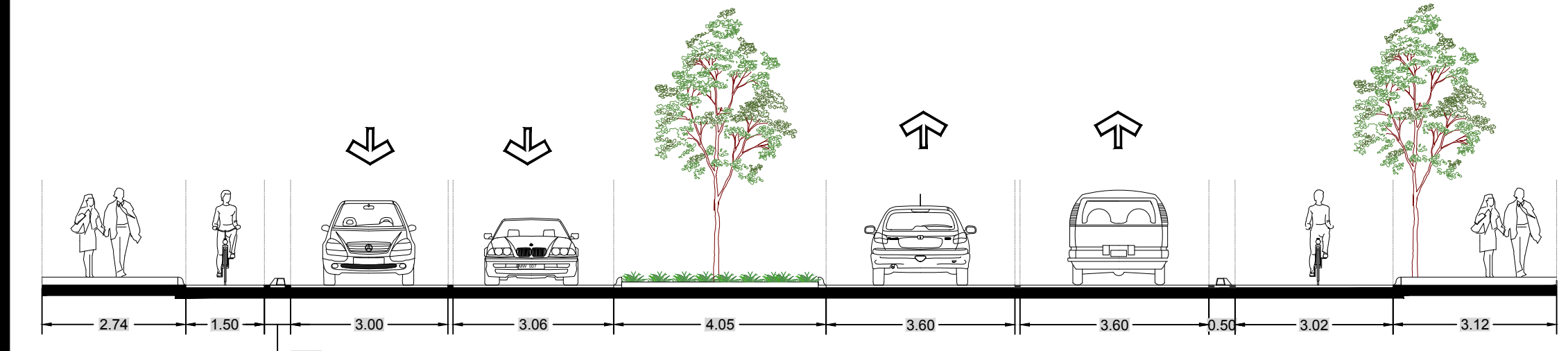
SECCIÓN DE CADENAMIENTO 1+200.00
